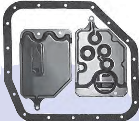
AISIN WARNER A240L-A244E Pan Gasket A240.GAS01 Filter A240.FIL01
