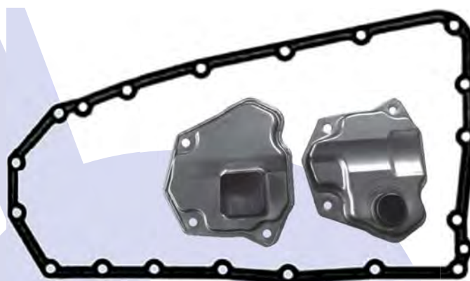
REOF10A (JF011E) (MITSUBISHI, CHRYSLER, NISSAN) Pan Gasket (18 Hole) JF011E.GAS01 Filter JF011E.FIL01 Cooler Return Filter JF011E.FIL02
