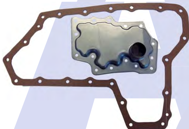
JATCO JF010E, NISSAN REOF09A (NISSAN MAXIMA & MURANO) Pan Gasket RE09.GAS01 Filter RE09.FIL01
