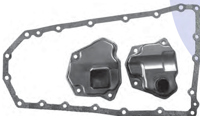
JATCO JF011E, NISSAN REOF10A (NISSAN) Pan Gasket (19 Hole) JF011E.GAS02 Filter JF011E.FIL01 Cooler Return Filter JF011E.FIL02
