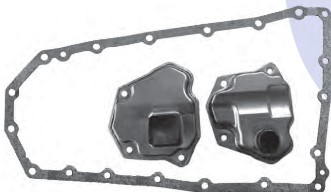
REOF10A (JF011E) (NISSAN) Pan Gasket (19 Hole) JF011E.GAS02 Filter JF011E.FIL01 Cooler Return Filter JF011E.FIL02
