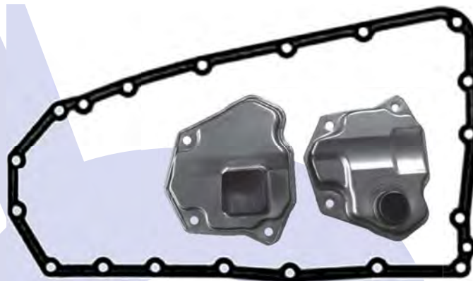
JATCO JF011E, NISSAN REOF10A (MITSUBISHI, CHRYSLER, NISSAN) Pan Gasket (18 Hole) JF011E.GAS01 Filter JF011E.FIL01 Cooler Return Filter JF011E.FIL02
