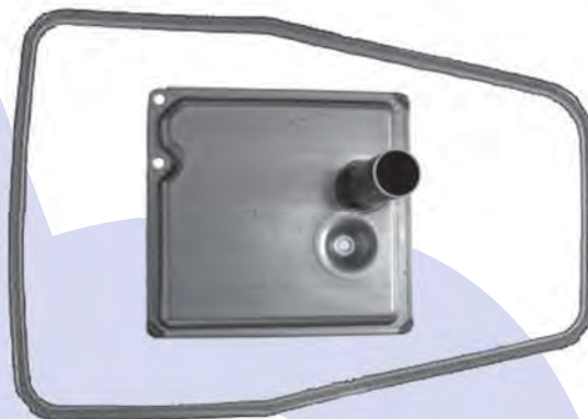
4HP24A CODE 1043 040 XXX Pan Gasket 4HP22.GAS08 Filter 4HP24A.FIL01
