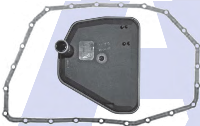
09L (6HP19AV) CODE 1071 014 XXX Pan Gasket 6HP19A.GAS01 Filter 6HP19A.FIL01
