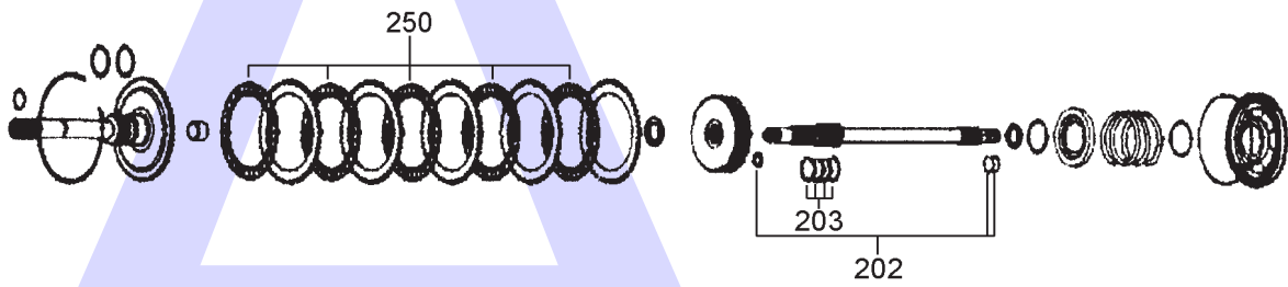
C1 Clutch
